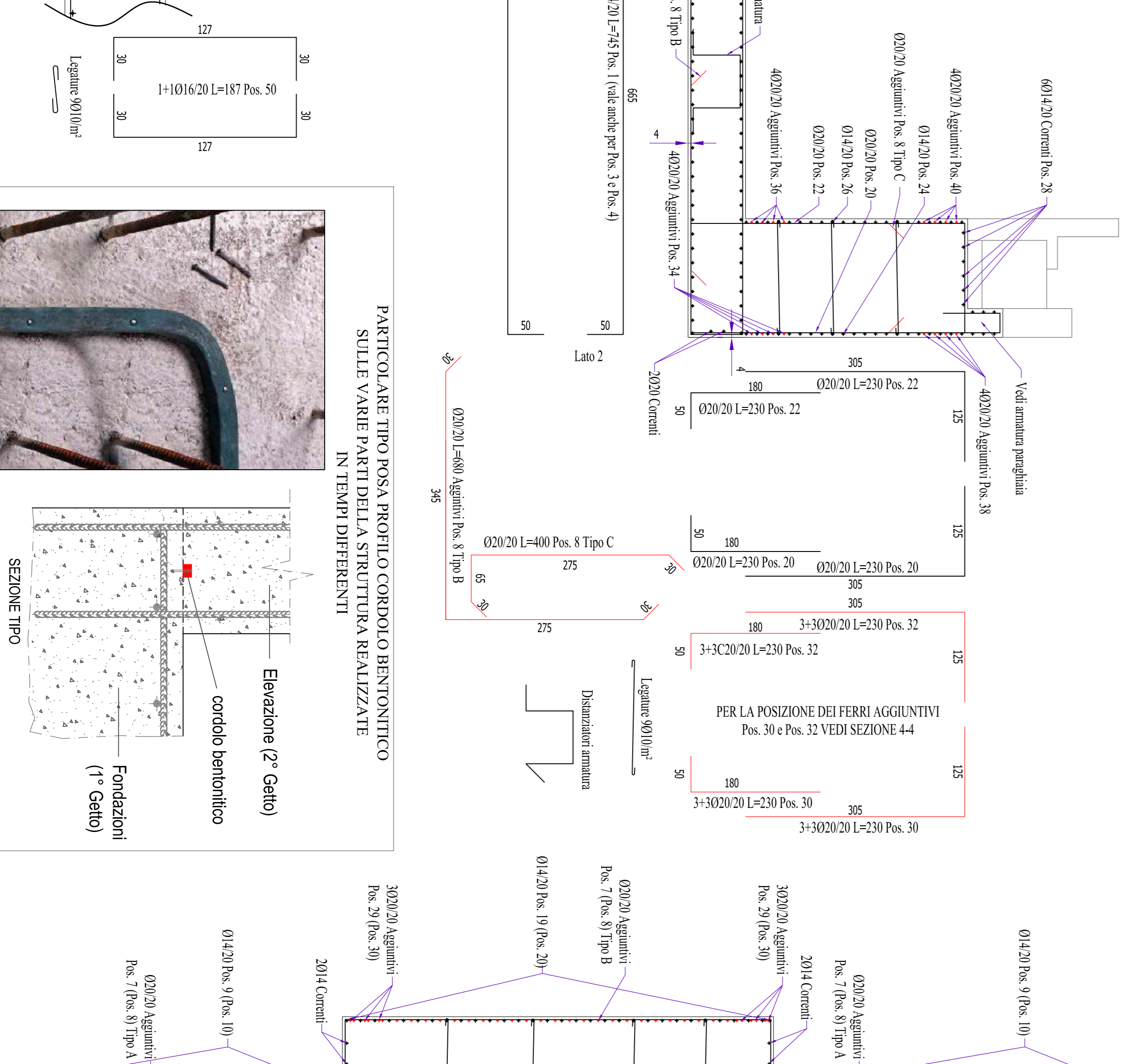
SEZIONE 3-3 DISTINTA ARMATURA PARETI FONDAZIONE - 1:50
